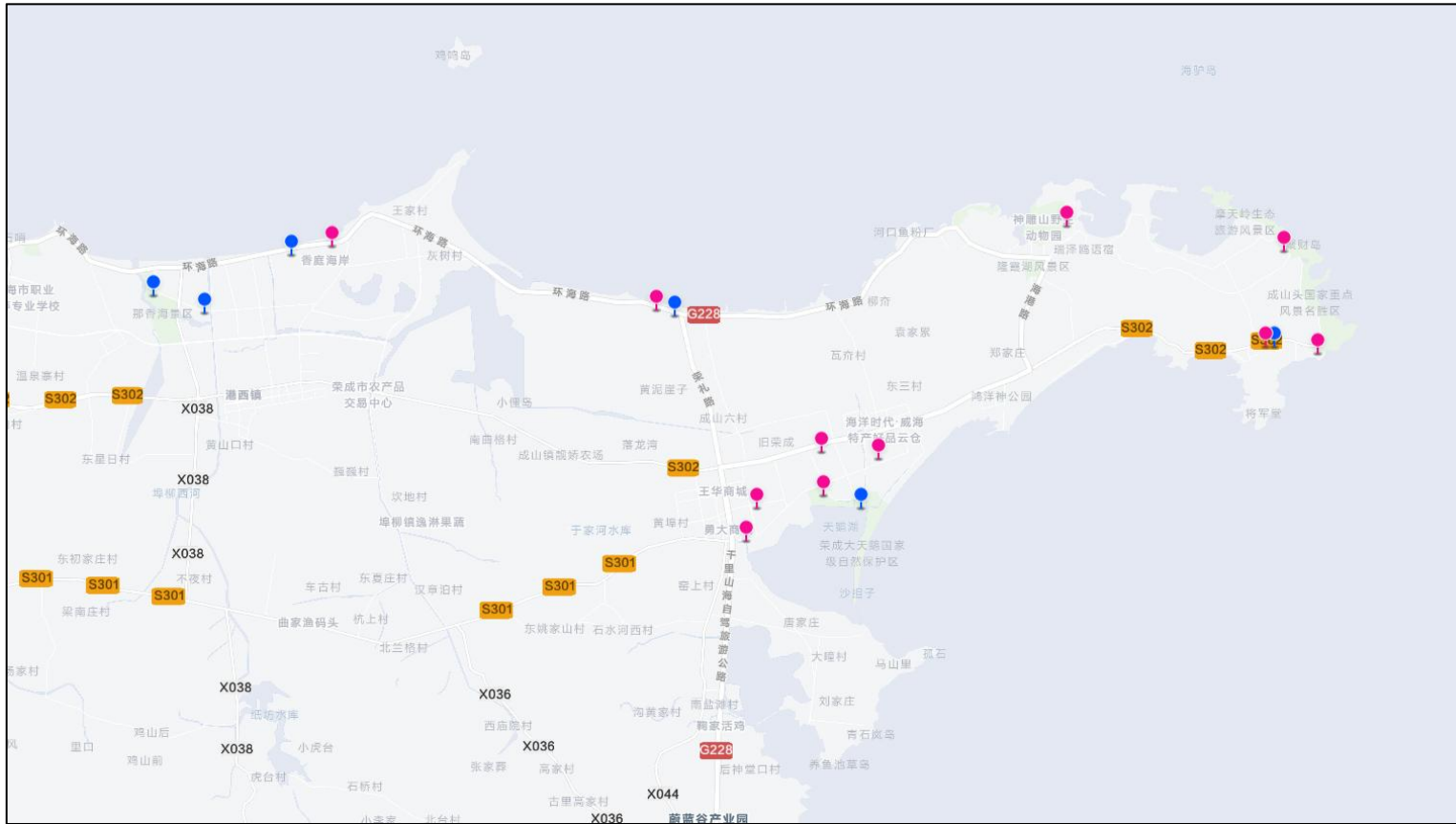
好运角旅游度假区充电站布局图
